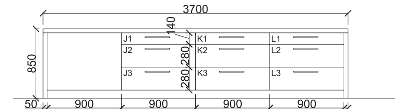
ELEVATION B
